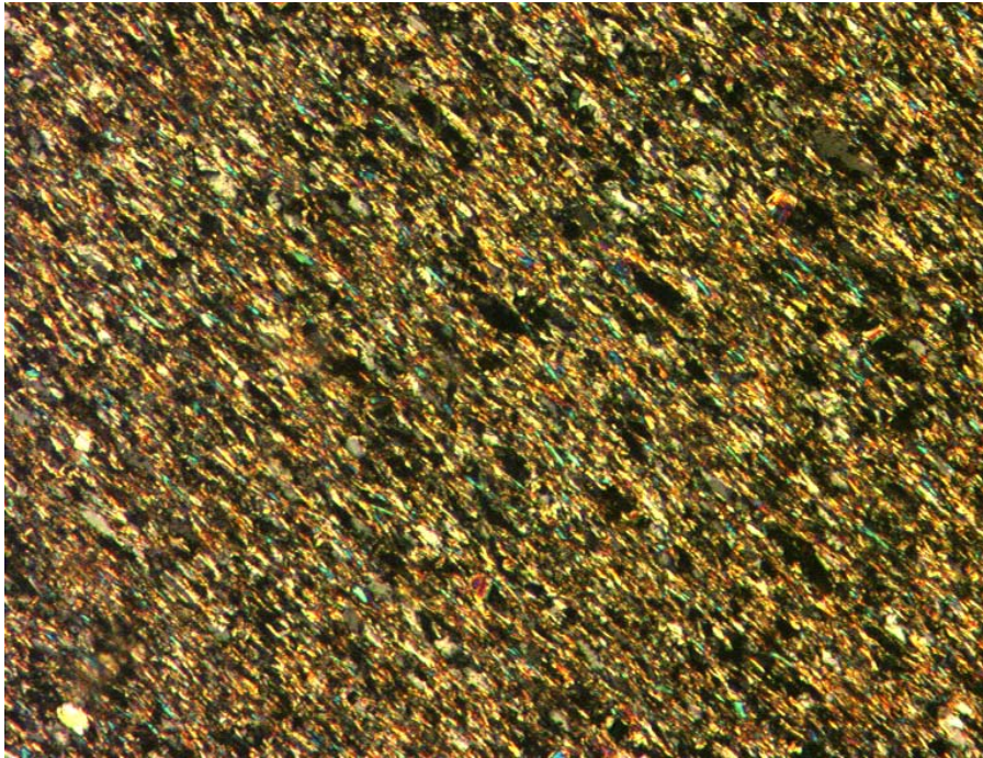
Bild 1: Ausschnitt aus der Probe Primero-Schiefer P83 (Schnitt senkrecht zur Schieferung), 100fache Vergrößerung, gekreuzte Polarisatoren, Aufnahme mit Texturanalysesystem
