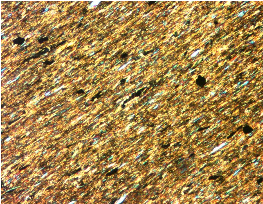
Bild 1: Ausschnitt aus der Probe Primero-Schiefer P14 (Schnitt senkrecht zur Schieferung), 100fache Vergrößerung, gekreuzte Polarisatoren, Aufnahme mit Texturanalysesystem
